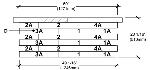
ELEVATION A
