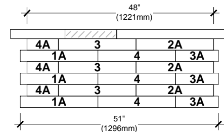
ELEVATION B
